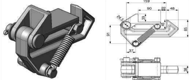
60014IT Kit mecanismo posterior 26 ton 000720
