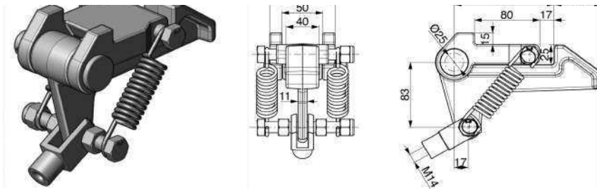
60014IT Kit mecanismo posterior 26 ton 000720
