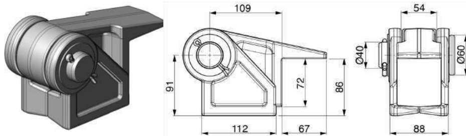
60036IT ARTICULAÇÃO REBATIVEL POST. GRANDE
