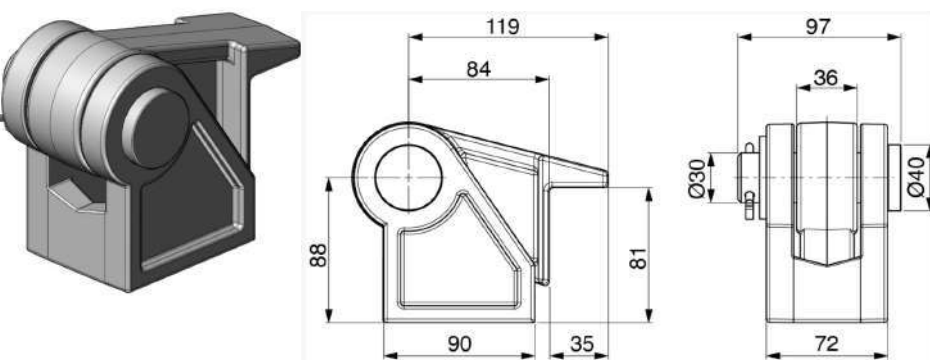
60043IT ARTICULAÇÃO REBATIVEL POST. GRANDE
